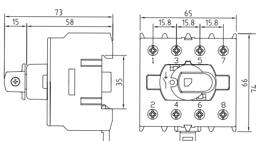
4-pólové provedení
