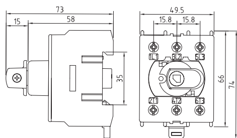
3-pólové provedení
